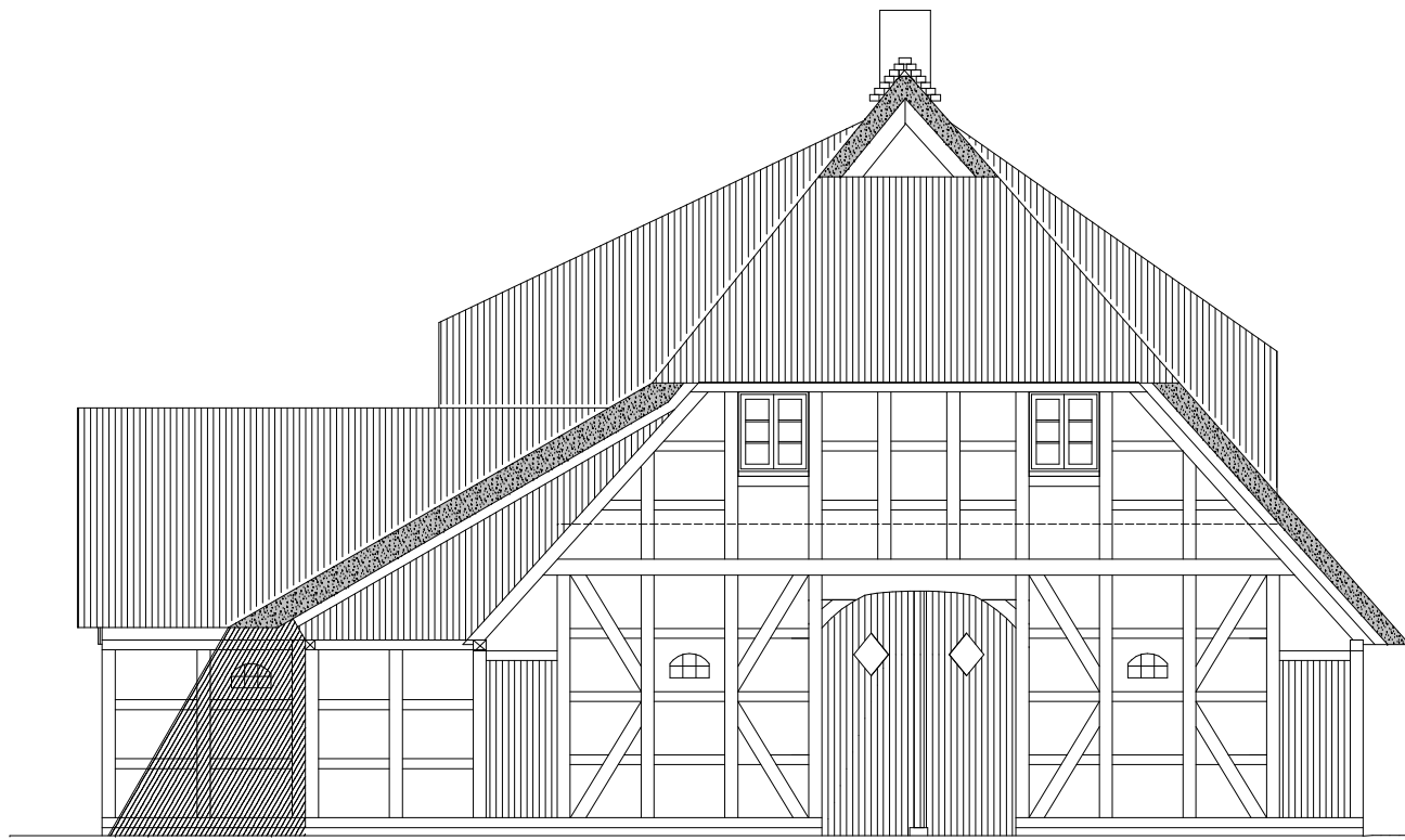
Ansicht West Entwurf/Ausführung
